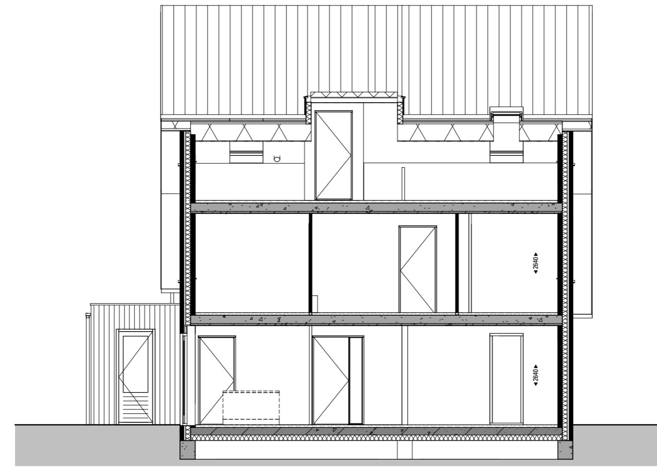
Dwarsnede B 1:100
