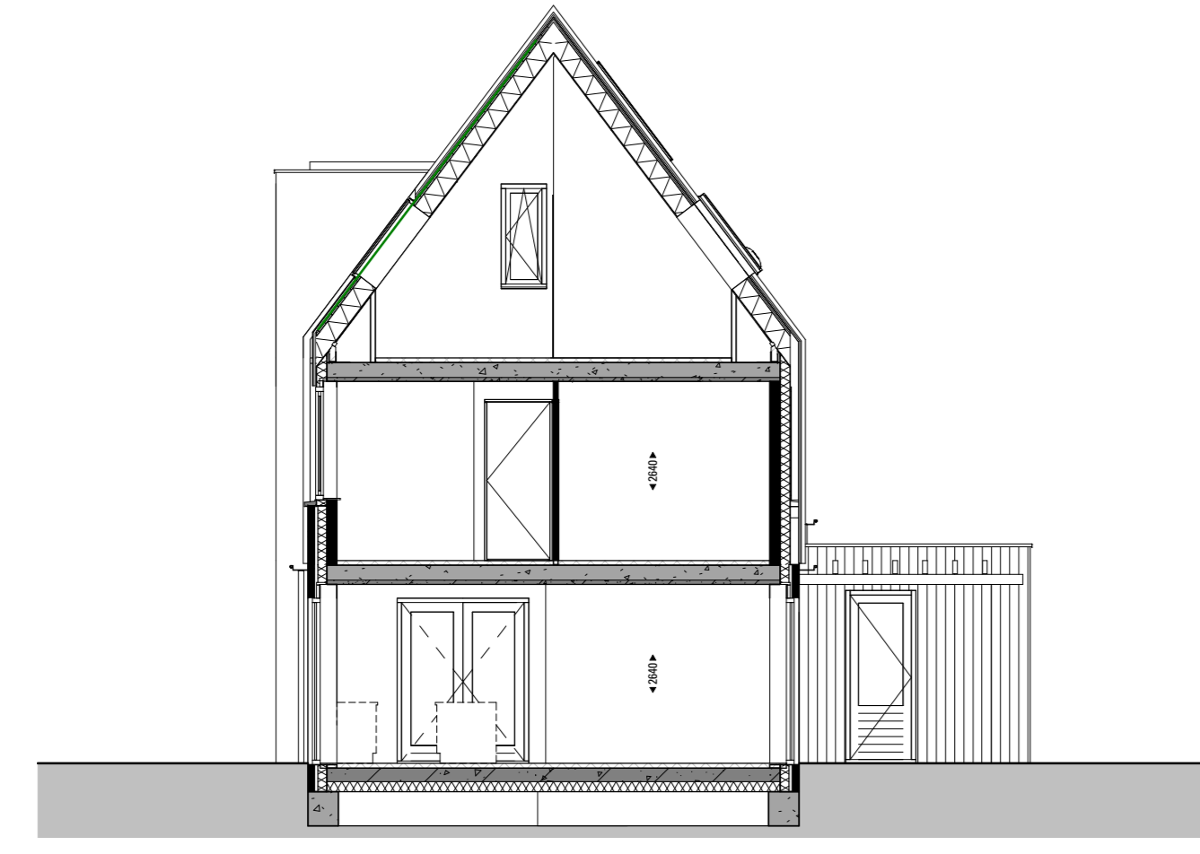
Dwarsnede A 1:100
