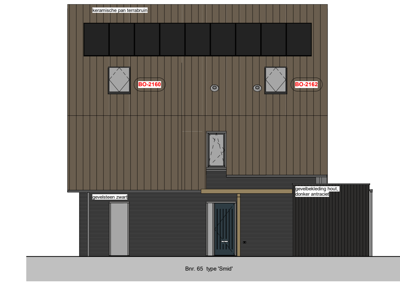
Rechterzijansicht 1:100
