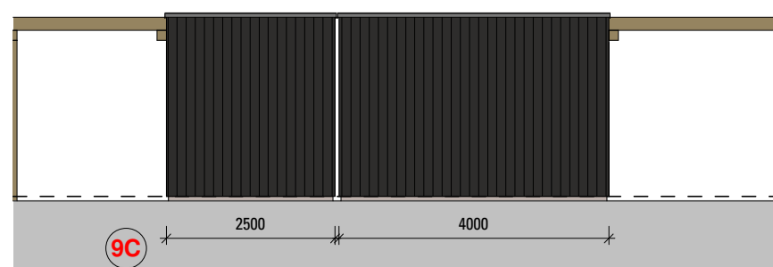
Aanzicht straatzijde 1:100
