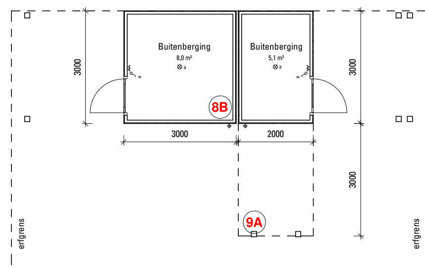
Begane grond tuinzijde 9A 1:100
