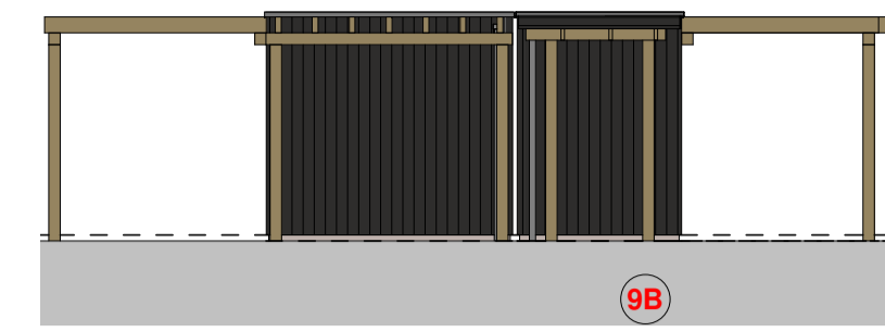
Aanzicht tuinzijde 1:100
