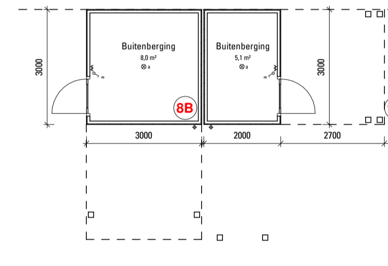
Begane grond 9D 1:100
