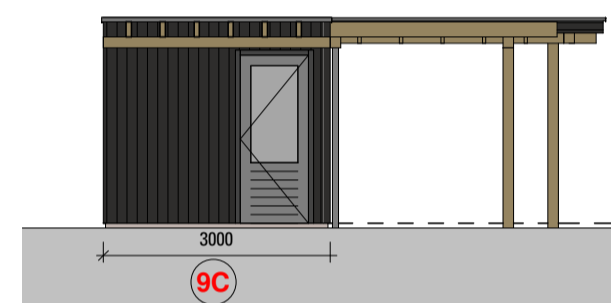
Linker zij aanzicht 1:100
