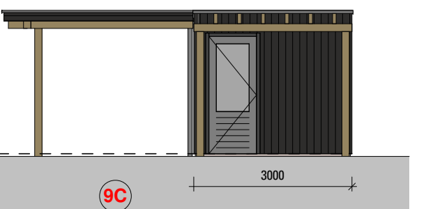
Rechter zij aanzicht 1:100
