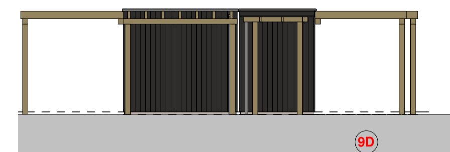
Aanzicht tuinzijde 1:100
