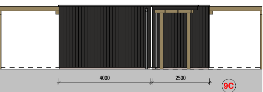
Aanzicht tuinzijde 1:100
