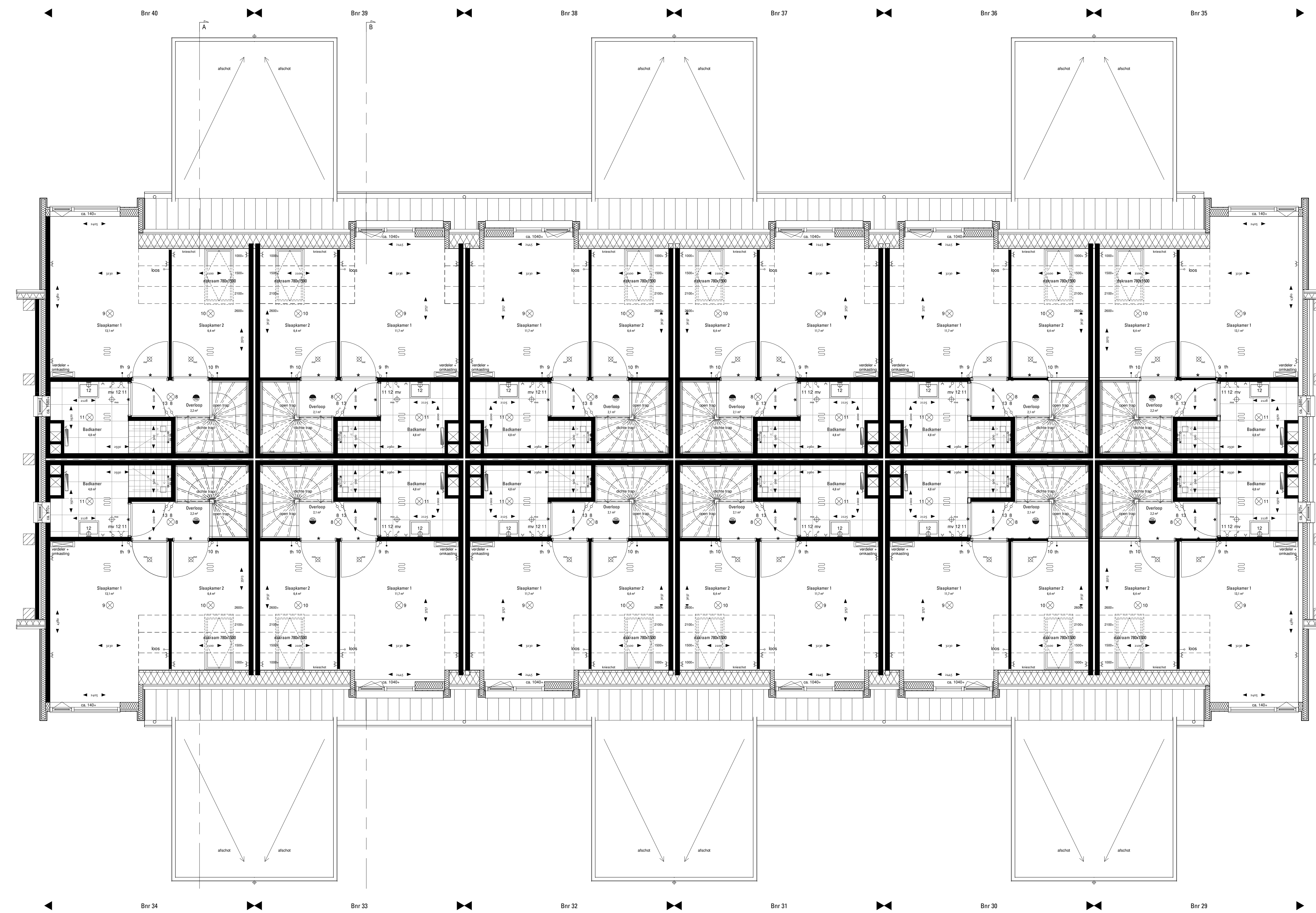
1e verdieping 1:50
