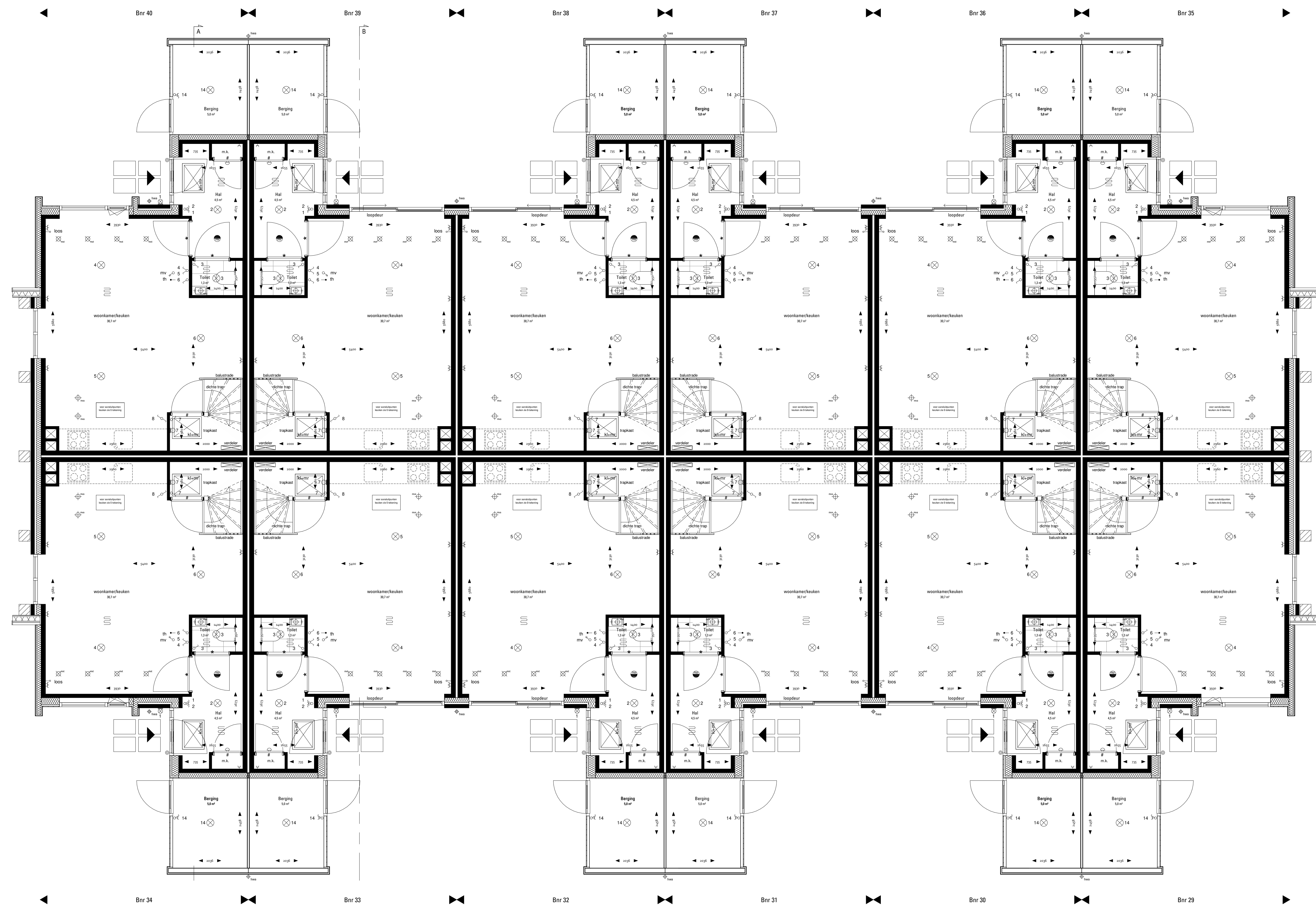
Begane grond 1:50
