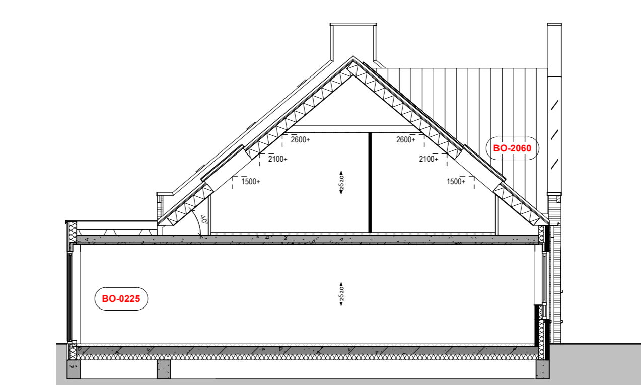
Doorsnede A3 1:100
