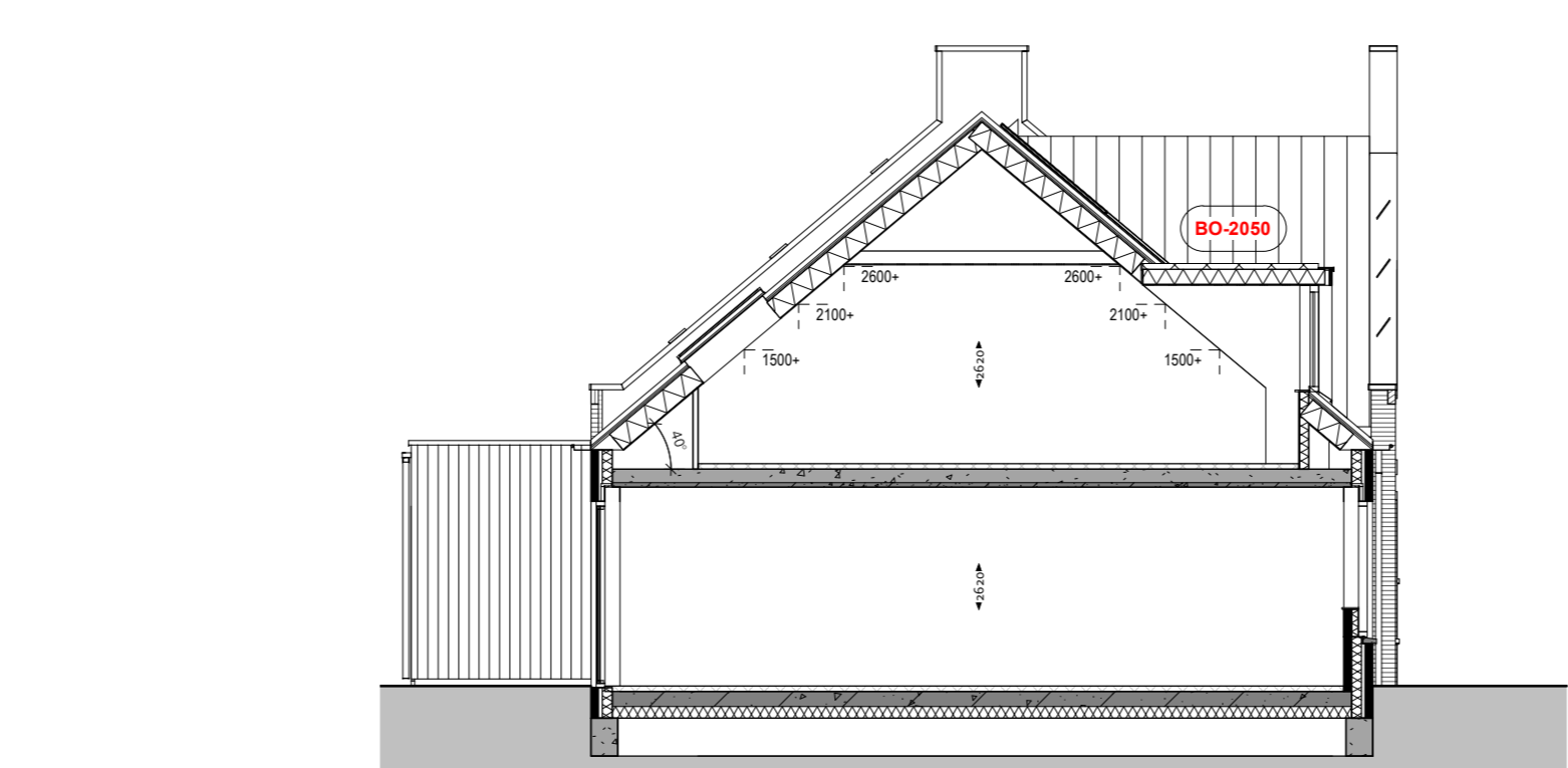
Doorsnede A1 1:100
