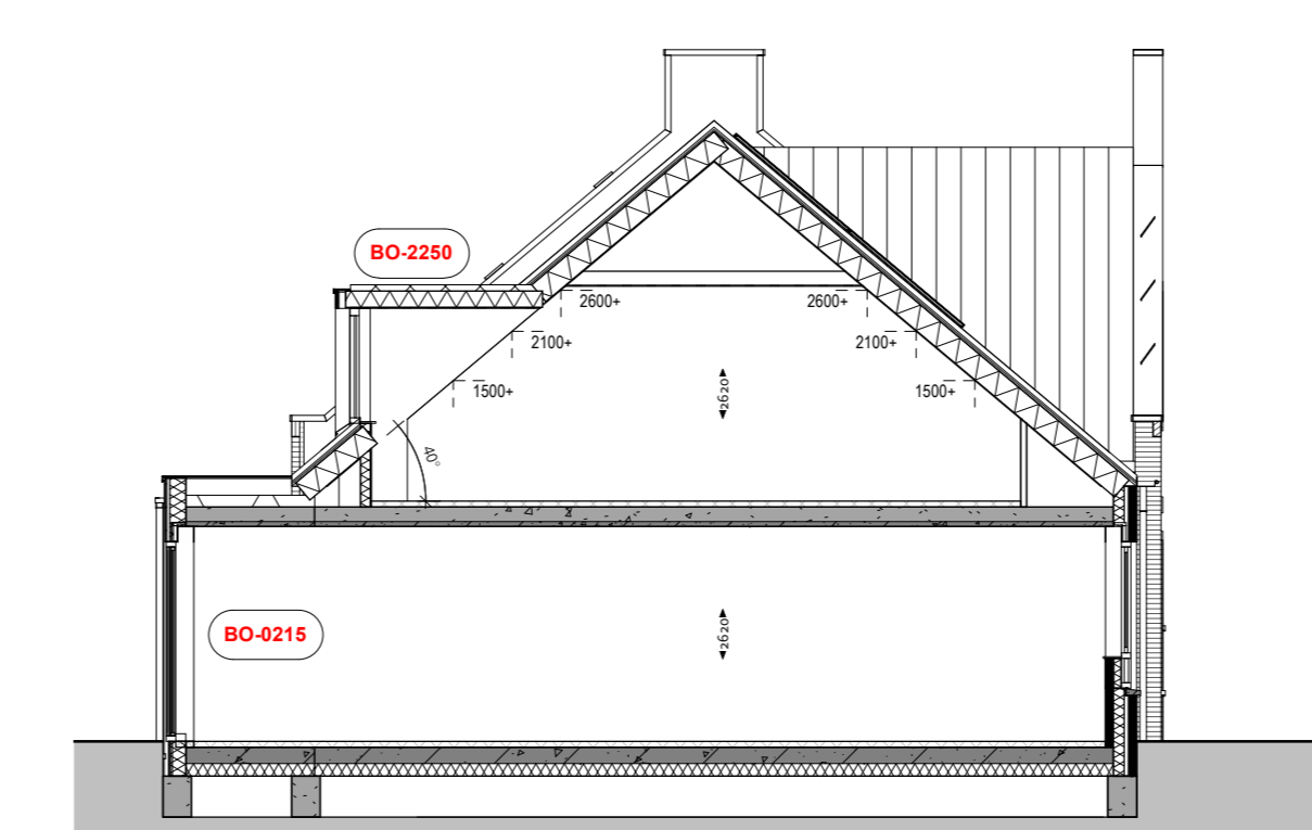
Doorsnede A2 1:100
