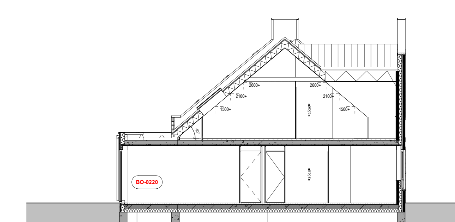
Doorsnede B1 1:100
