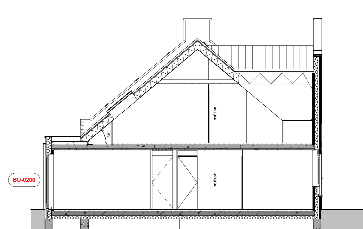
Doorsnede B2 1:100
