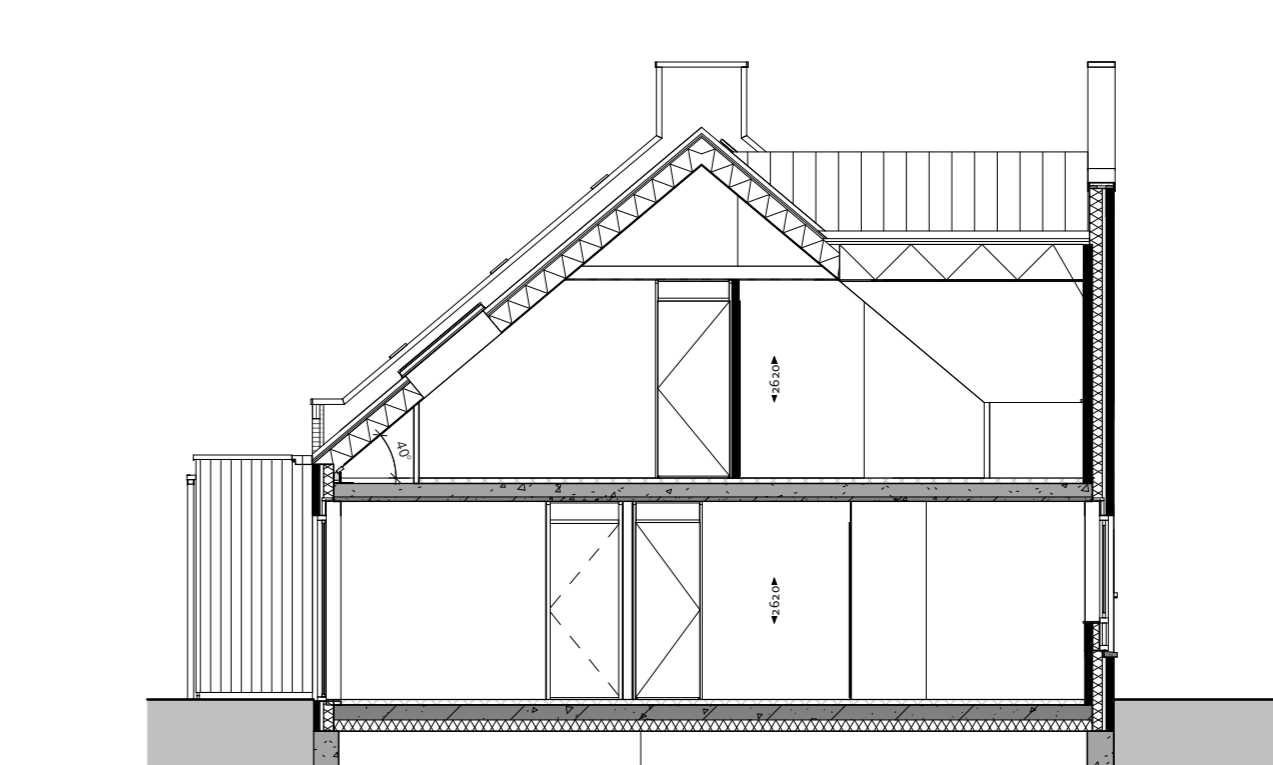
Doorsnede B3 1:100
