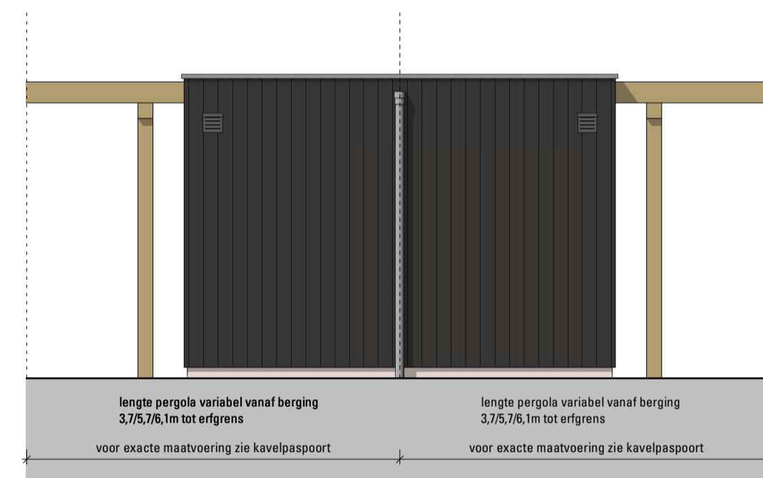
Aanzicht tuinzijde 1:50
