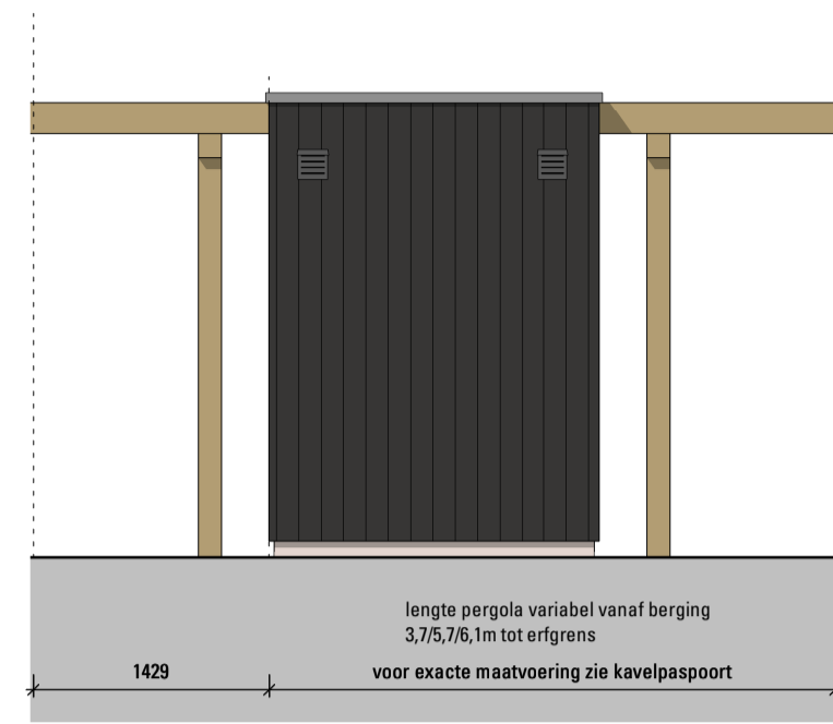
Aanzicht straatzijde 1:50
