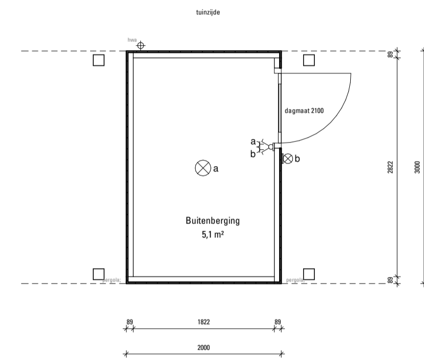
Begane grond 1:50
