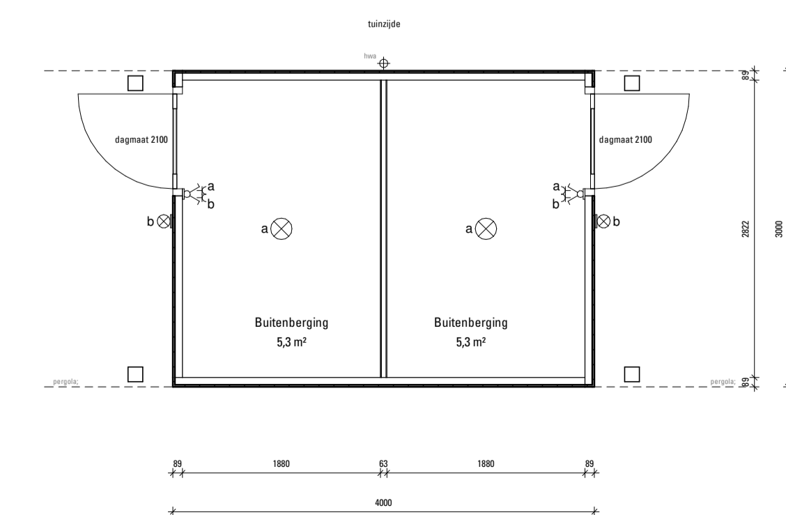
Begane grond 1:50
