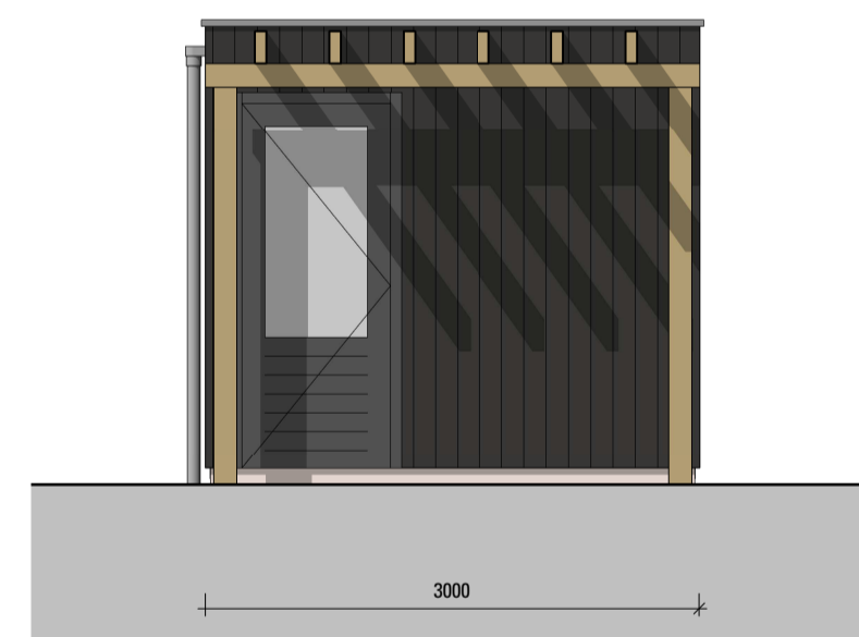
Linkerzijzicht 1:50
