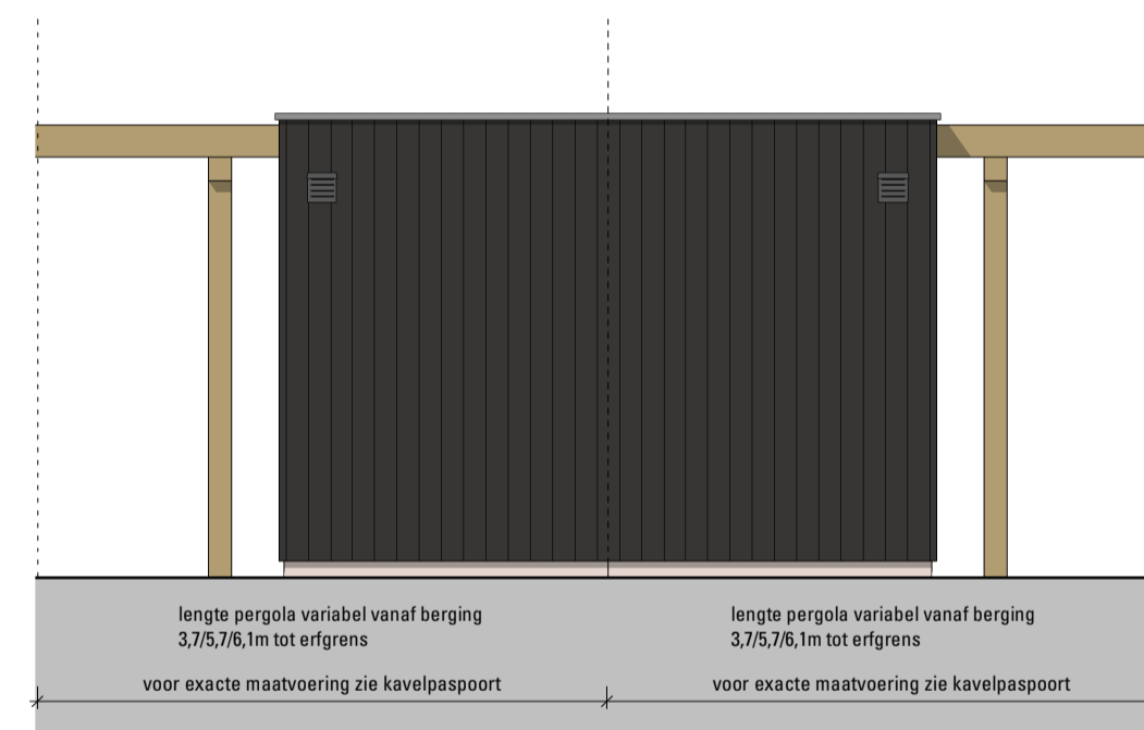
Aanzicht straatzijde 1:50
