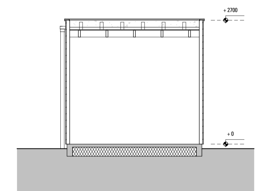
Doorsnede 2 1:50
