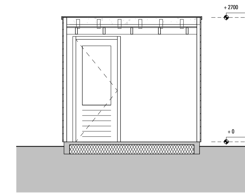
Doorsnede 1 1:50
