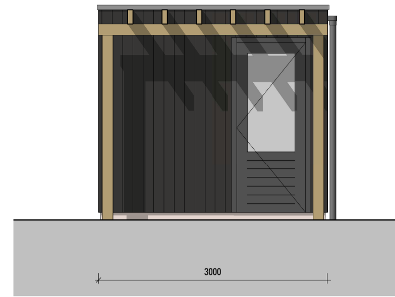
Rechterzijzicht 1:50
