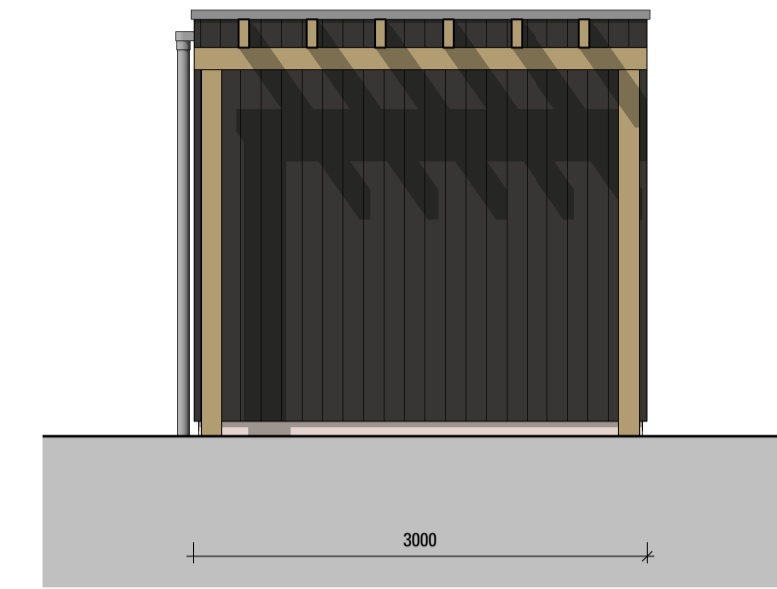
Linkerzijzicht 1:50
